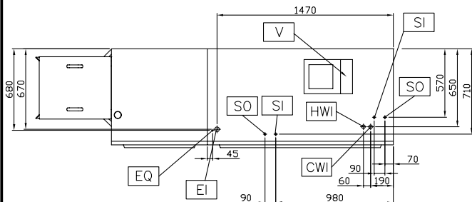
Boven aanzicht
